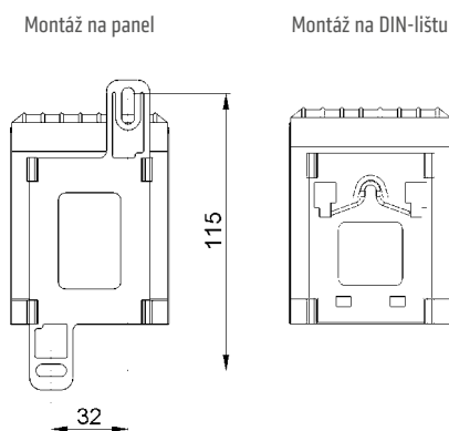
Pohled zezadu
